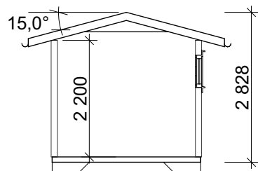
Snitt A-A
