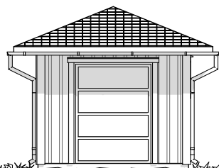
Fasade 1
