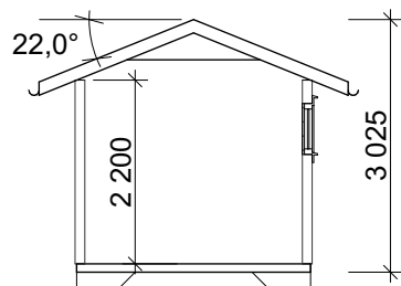
Snitt A-A
