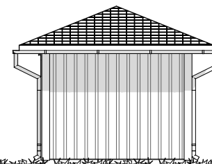
Fasade 3
