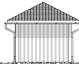
Fasade 3
