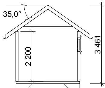
Snitt A-A
